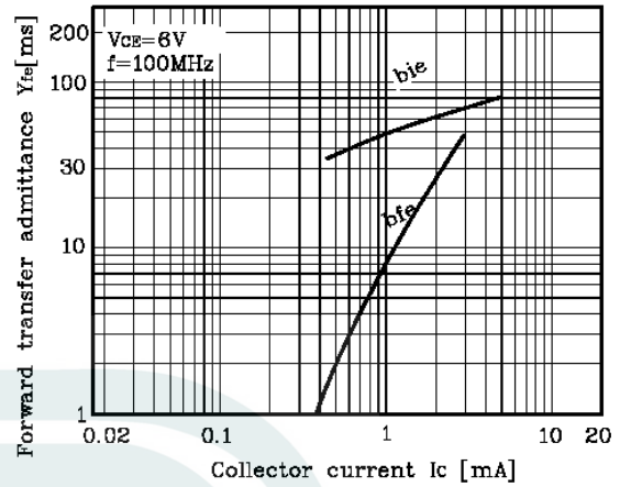
Fig. 8 I_C - Y_{fe}
